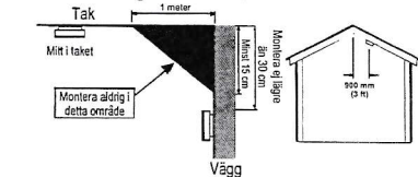
FIGUR 3i – Placering av brandvarnaren
