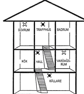
FIGUR 2 – FLERVÅNINGSBOSTAD
